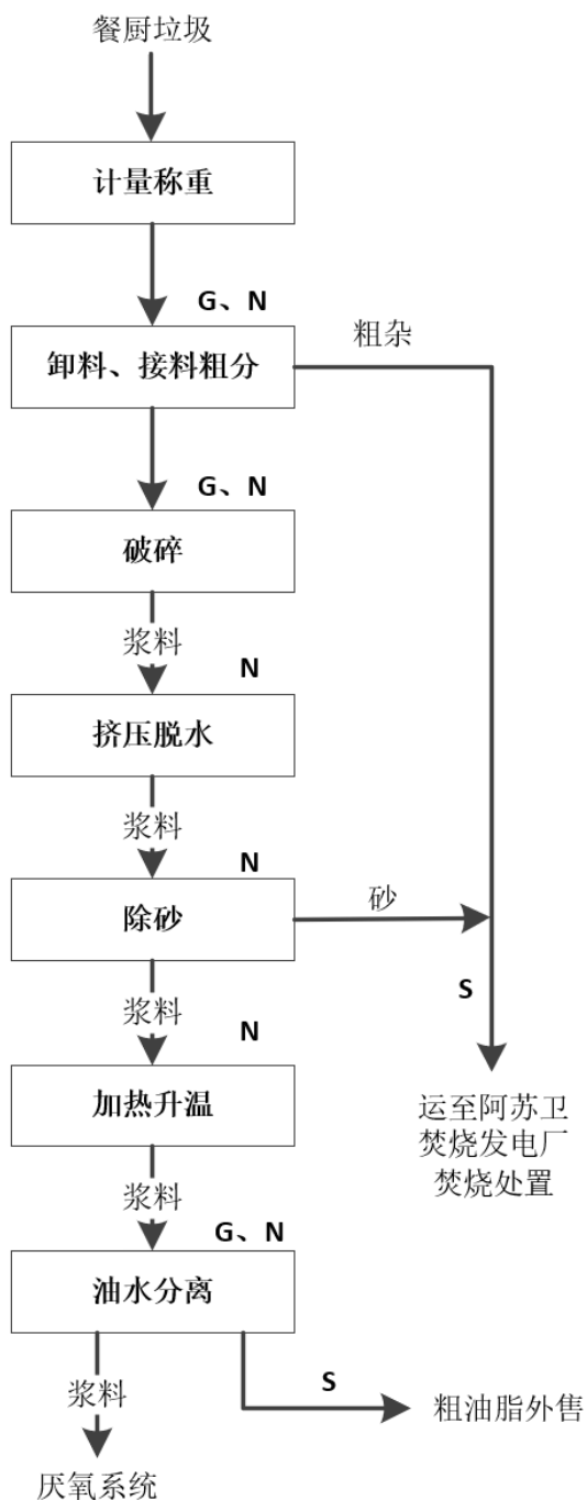
图 3-3 餐厨垃圾预处理系统工艺流程图
