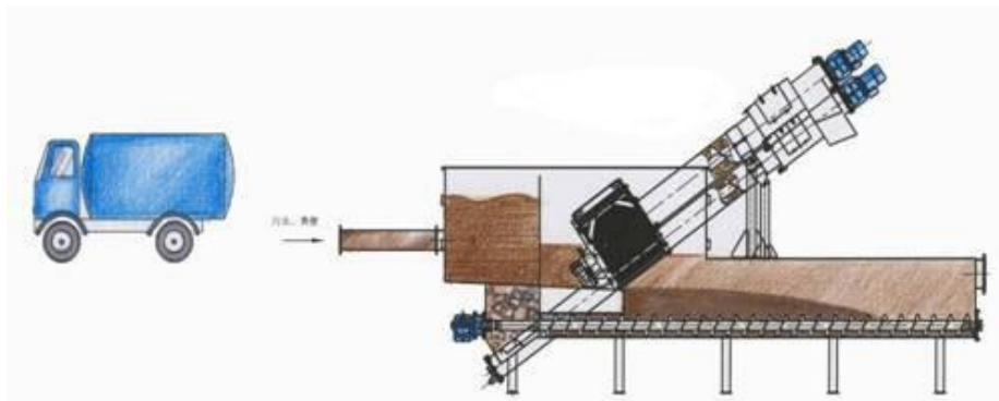
图 3-6 固液分离装置
