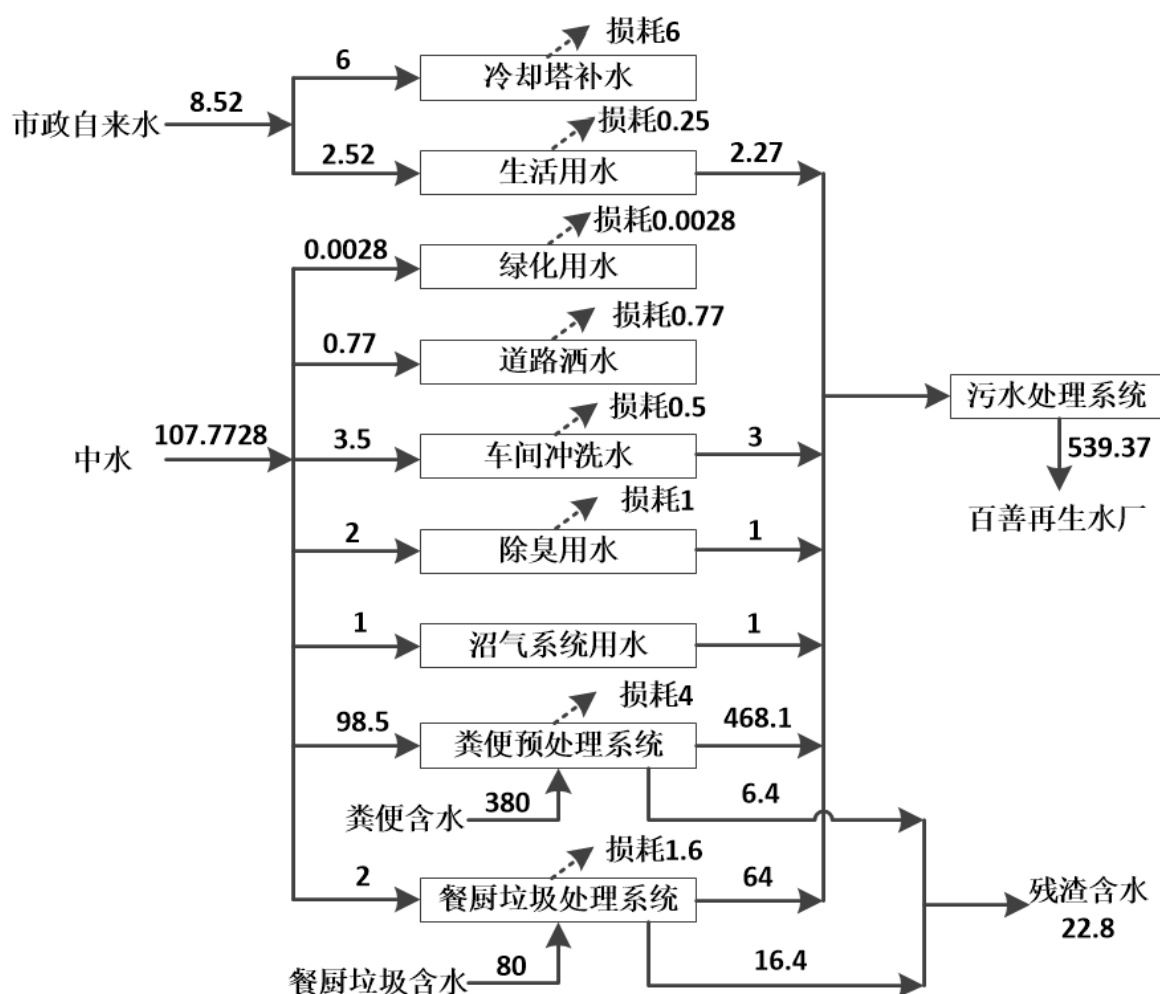
图 3-12 水平衡图 ( \text{m}^3/\text{d} )
