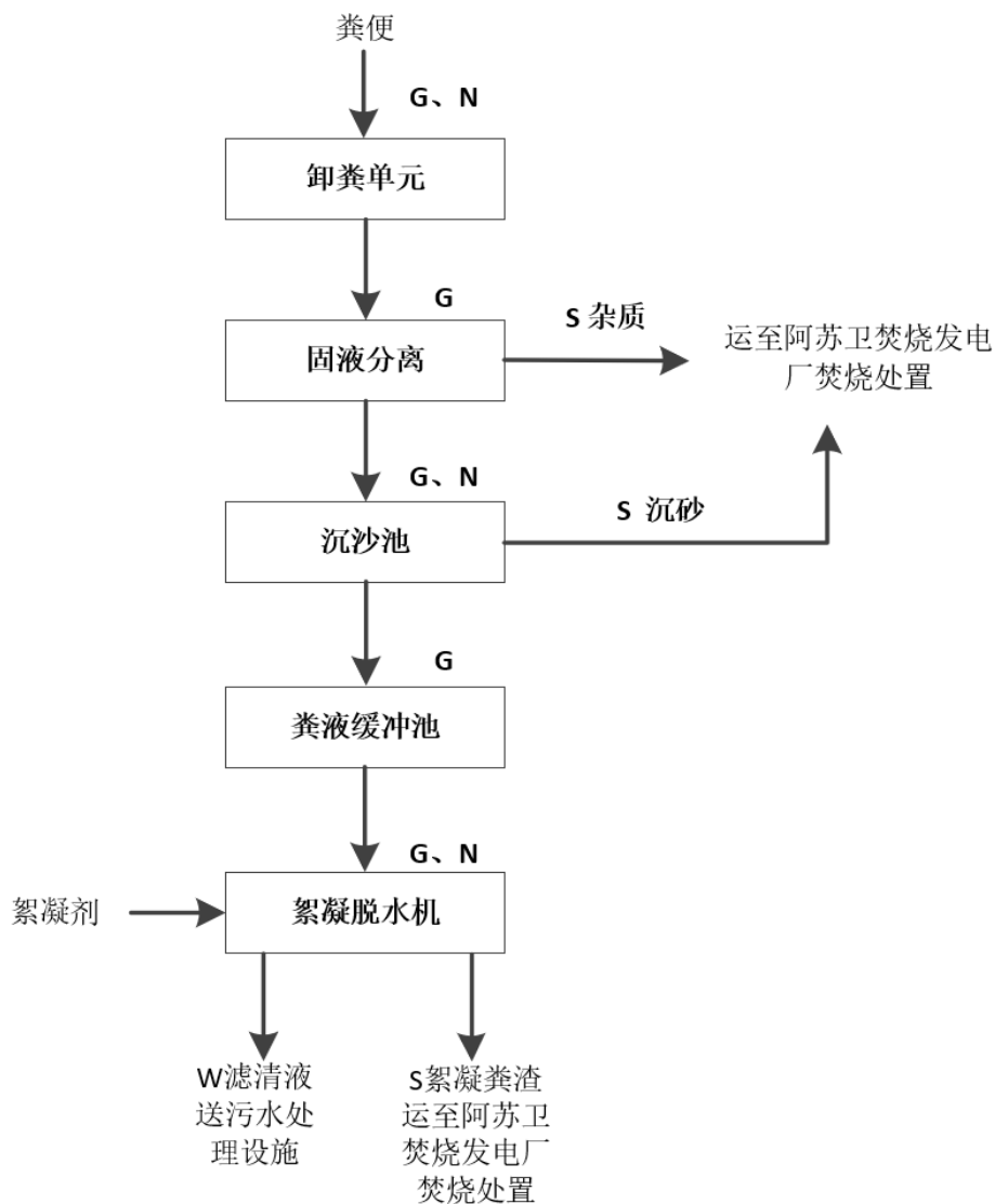
图 3-5 粪便预处理系统工艺流程图
