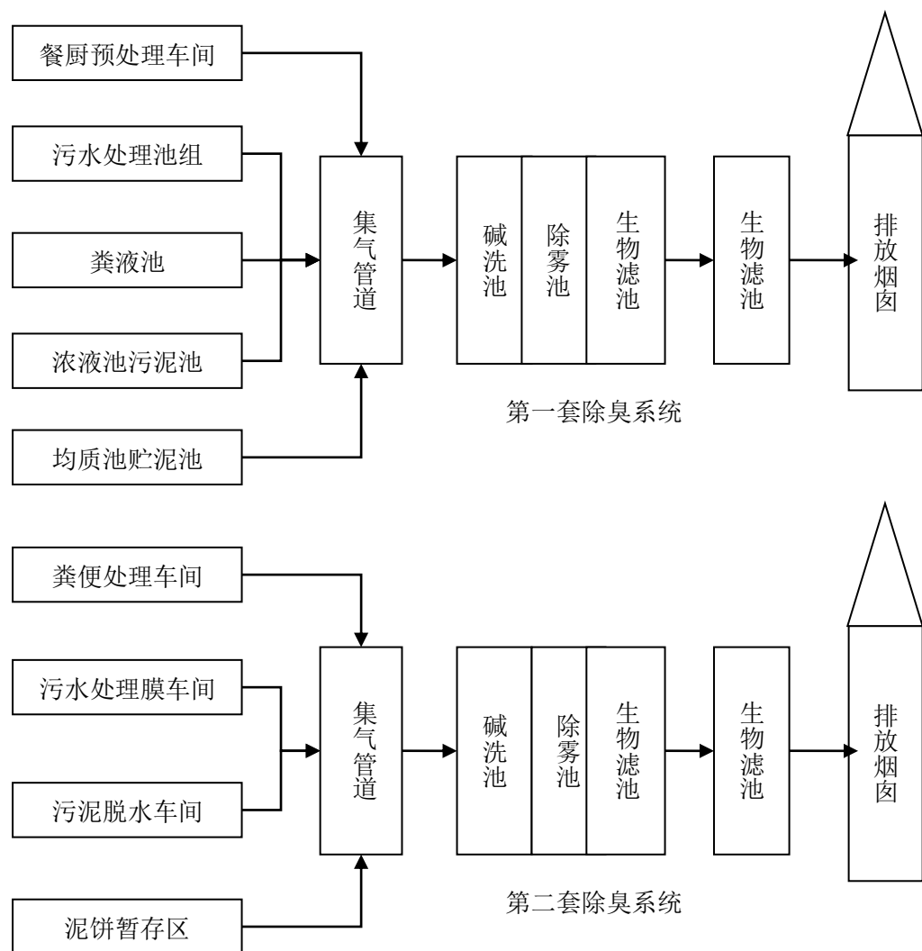
图 3-11 除臭工艺流程图
