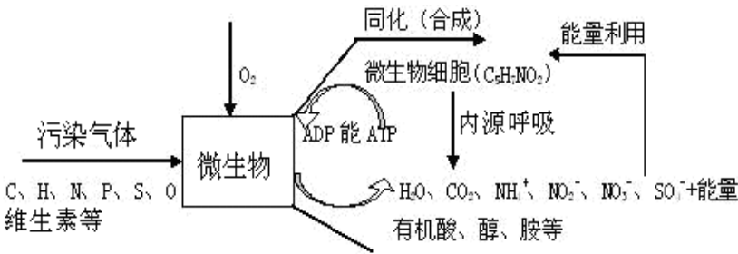
图 11-2 污染物转化机理图
