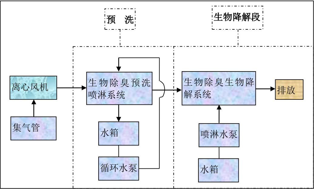
图 11-3 生物除臭工艺流程图
