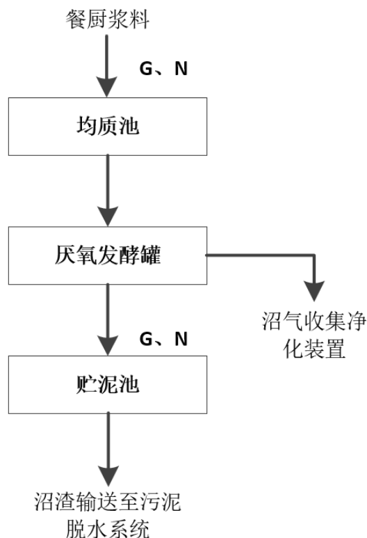
图 3-4 厌氧处理系统工艺流程图
