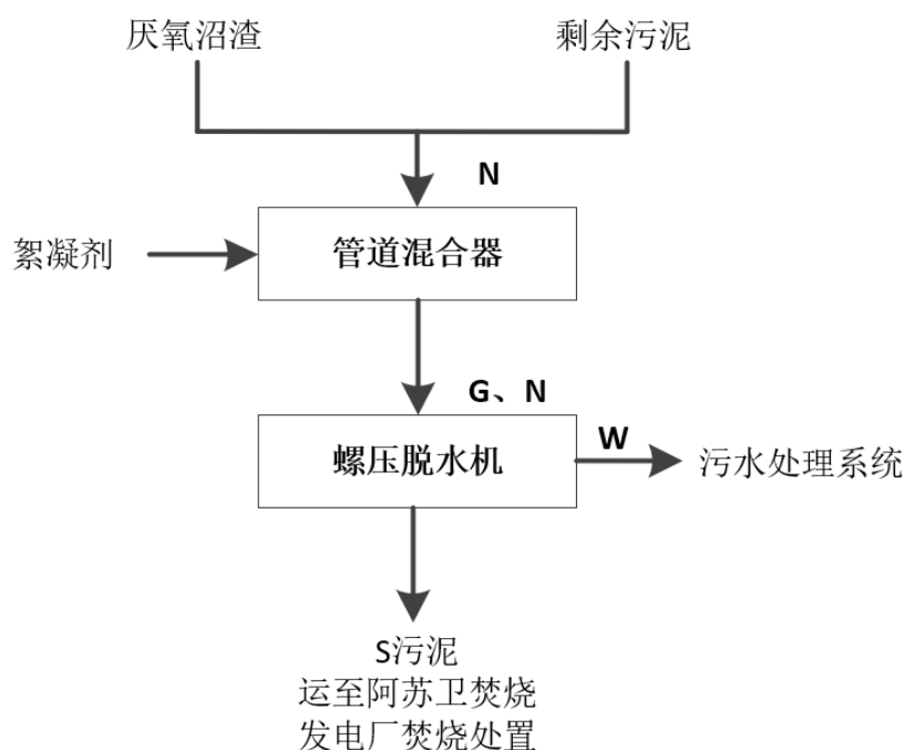
图 3-8 污泥脱水系统工艺流程图
