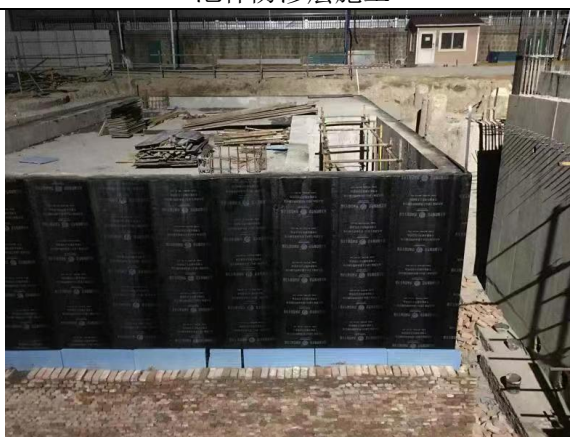
污水处理站
