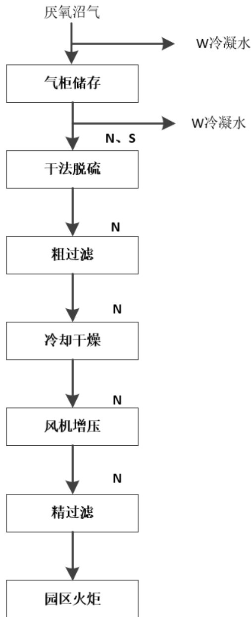
图 3-9 沼气净化存储系统工艺流程图
